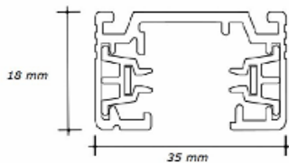
1-fase rail
